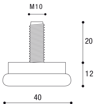
Scivolo metallico a vite Metal slider with screw
