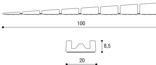
Spessore a cuneo (8 settori) Wedge in 8 sections
