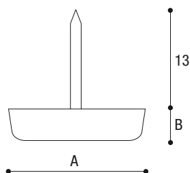
Scivolo Pratic Pratic slider
