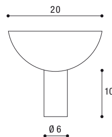
Ventosa per cristalli Suction cap for glass
