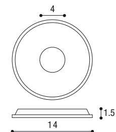
Rondella Washer
