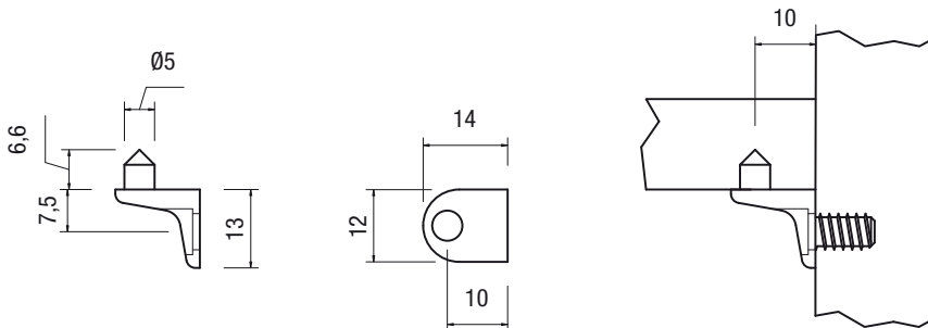
Con foro Ø 5 per vite With hole Ø 5 for screw
